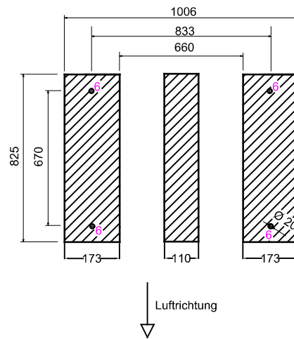
Draufsicht Sockel
